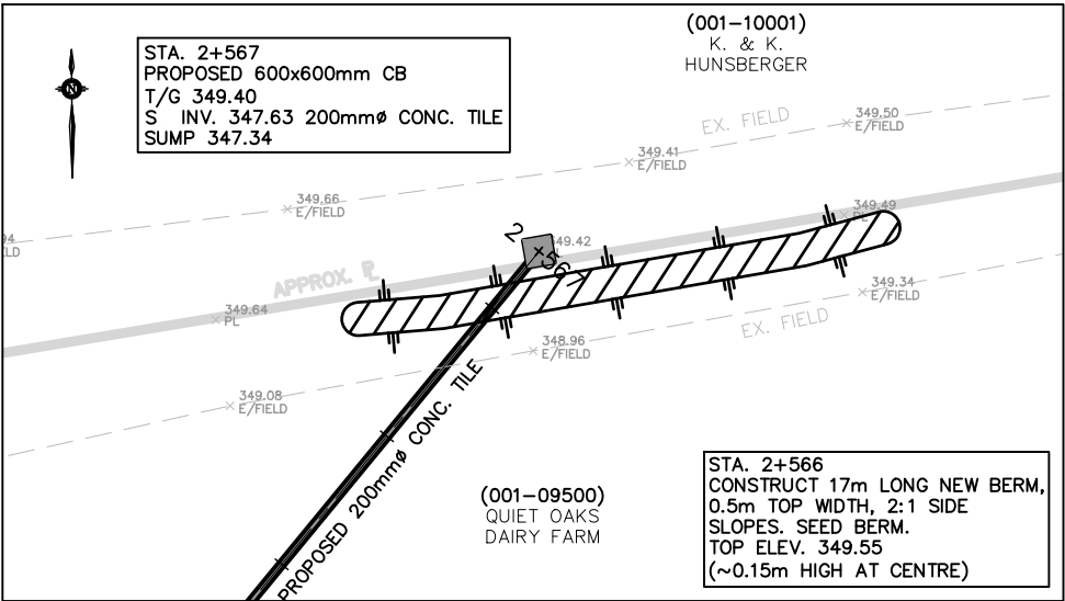
STA. 2+567: DETAIL
