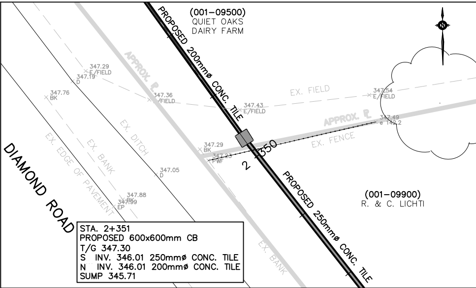
STA. 2+351: DETAIL
