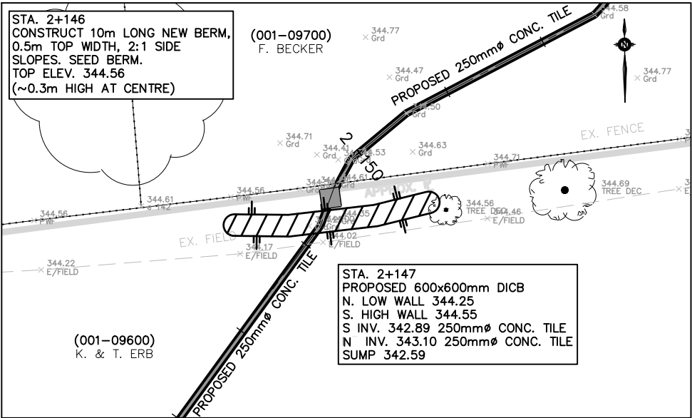
STA. 2+147: DETAIL
